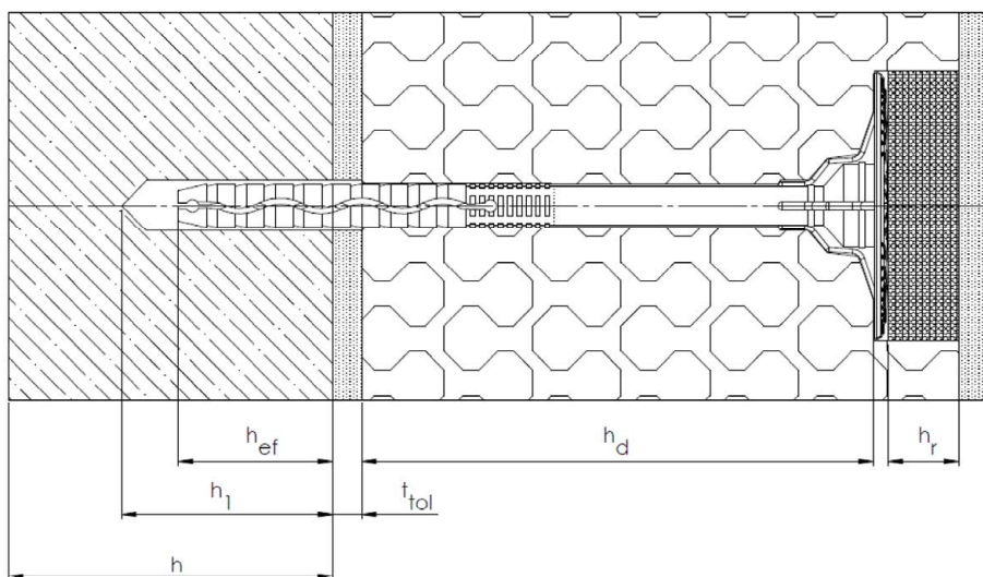
VERSENKTE MONTAGE
